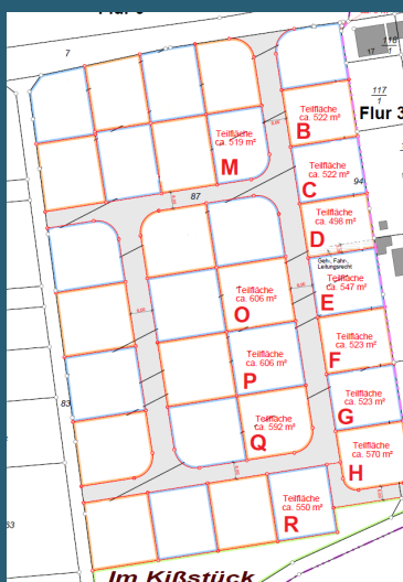
Foto / Bemaßungsskizze
