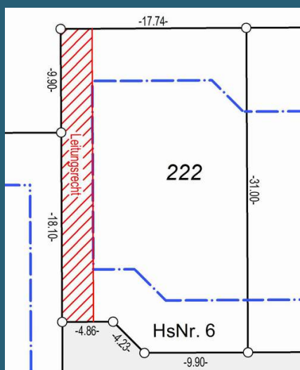
Foto / Bemaßungsskizze
