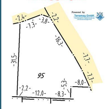
Foto / Bemaßungsskizze
